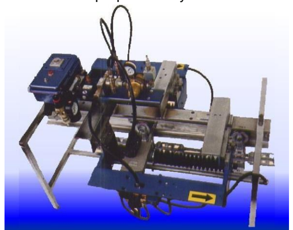
OP-201 mazání plastickým mazivem válečků hnacího řetězu
