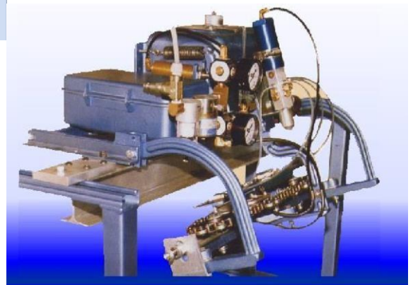
OP-4 mazání přepravníkových řetězů
