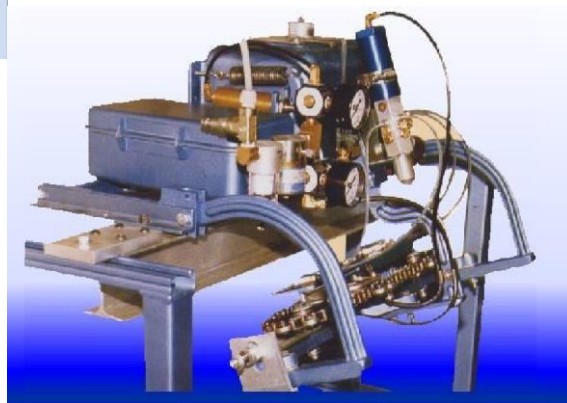
OP-4 смазка цепей транспортера
