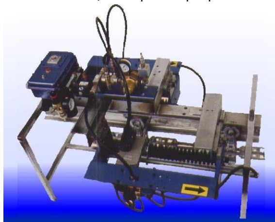
OP-201 смазка пластичной смазкой роликов ведущей цепи
