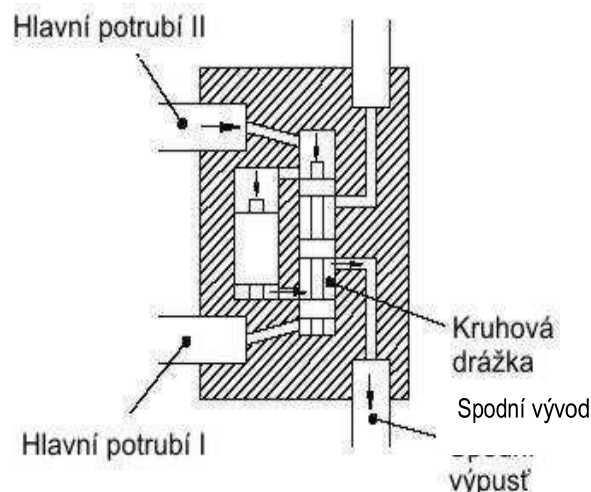
Pístový rozdělovač - takt 2
