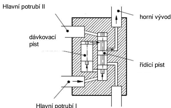
Pístový rozdělovač 1
