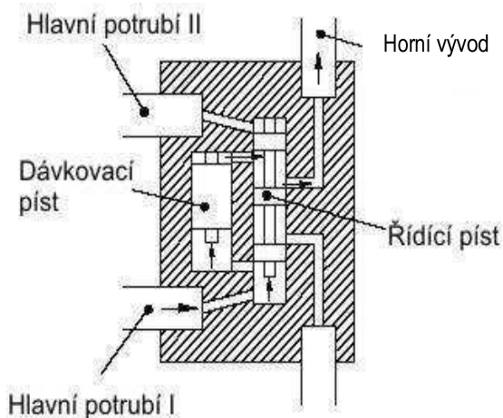
Pístový rozvaděč - takt 1
